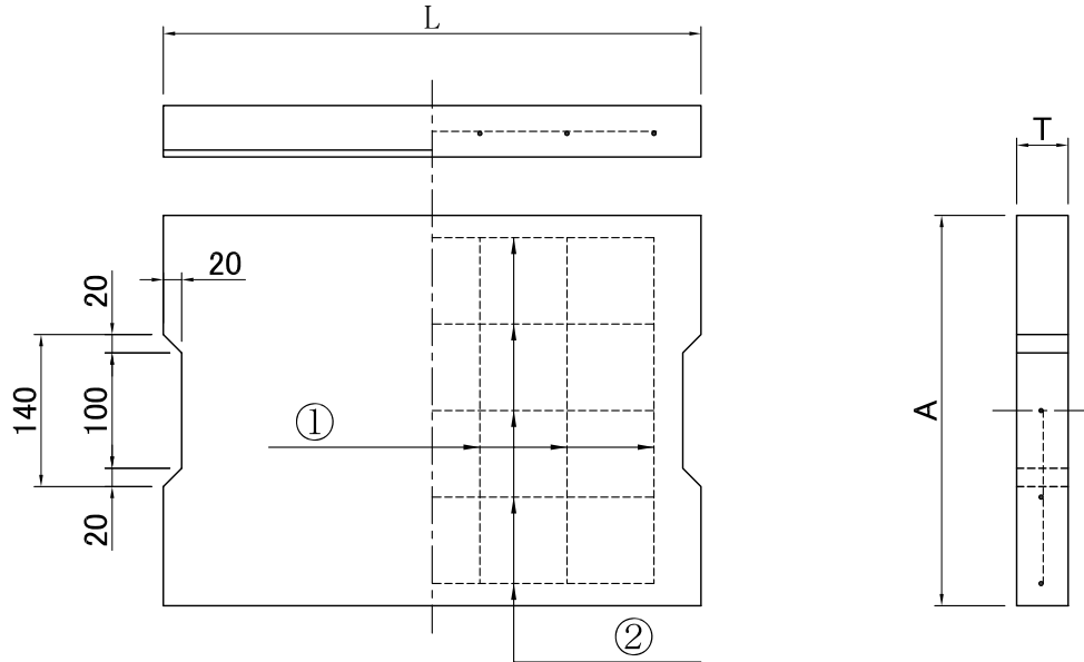
規格寸法表
